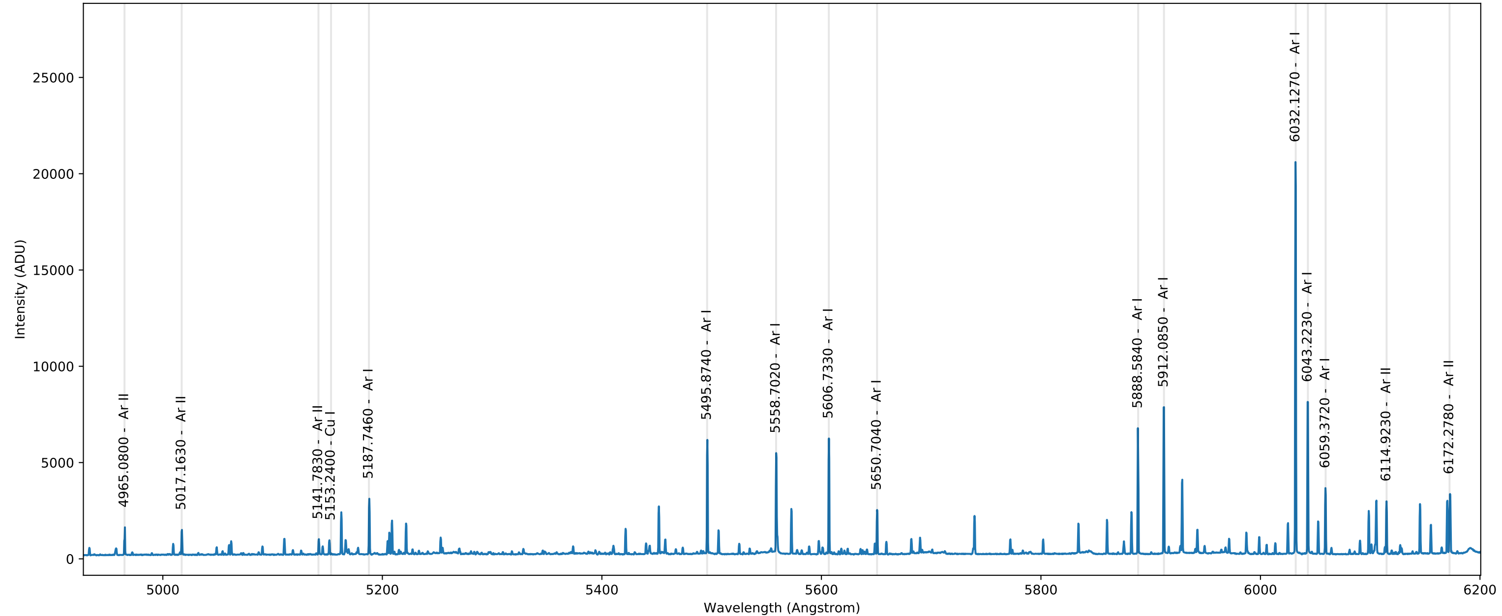
FeHeAr - 1200 m3
